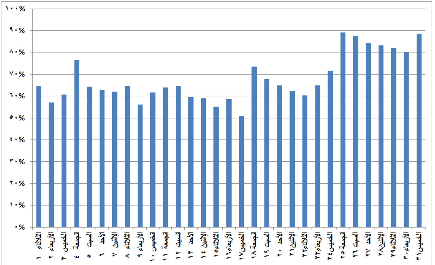
شكل (٢٨) نسب الفائض للحمل الاقصى المسجل يوميا خلال شهر أكتوبر ٢٠١٩
