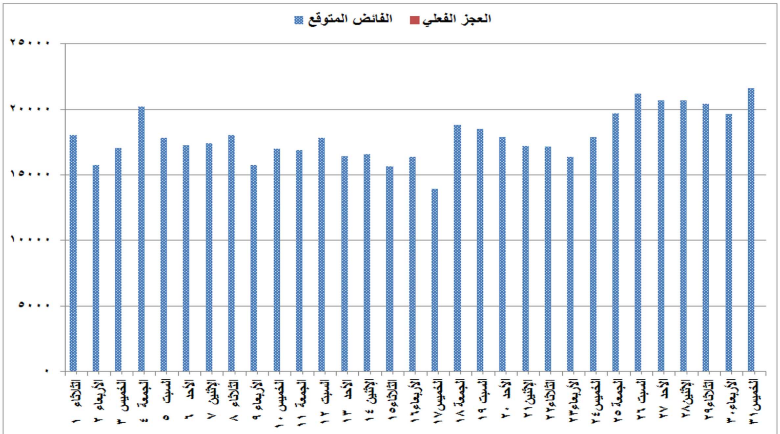
شكل (٧) الفائض والعجز المتوقع للقدرات خلال شهر أكتوبر ٢٠١٩
