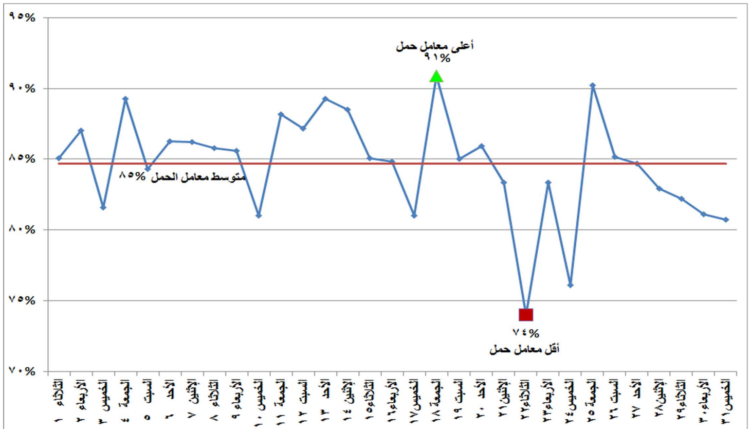
شكل (١٢) إجمالي معامل الحمل لوحدات الانتاج خلال شهر أكتوبر ٢٠١٩
