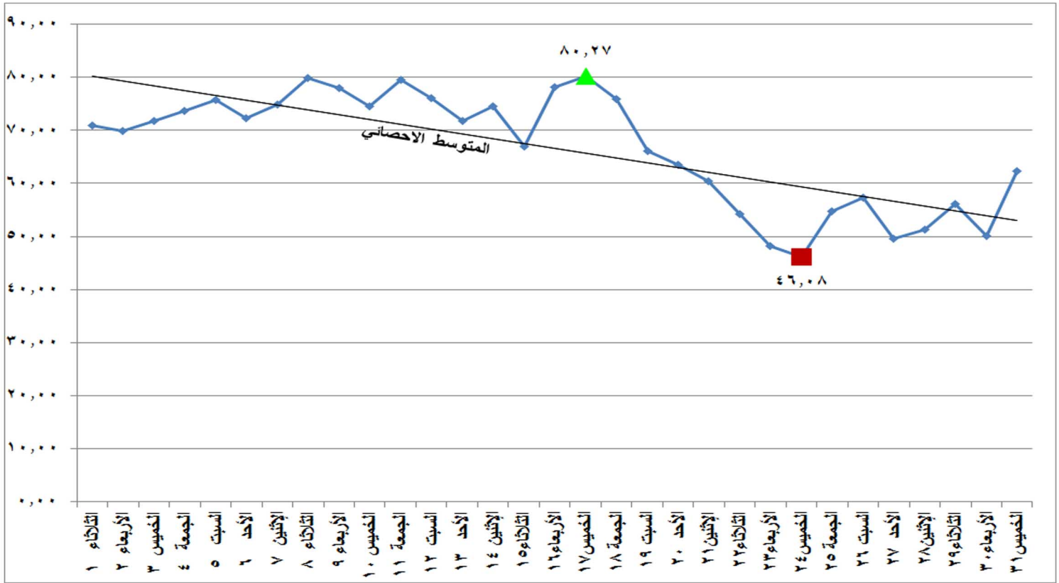
شكل (٢١) الطاقة الكهربائية المنتجة من المصادر غير الحرارية خلال شهر أكتوبر ٢٠١٩
