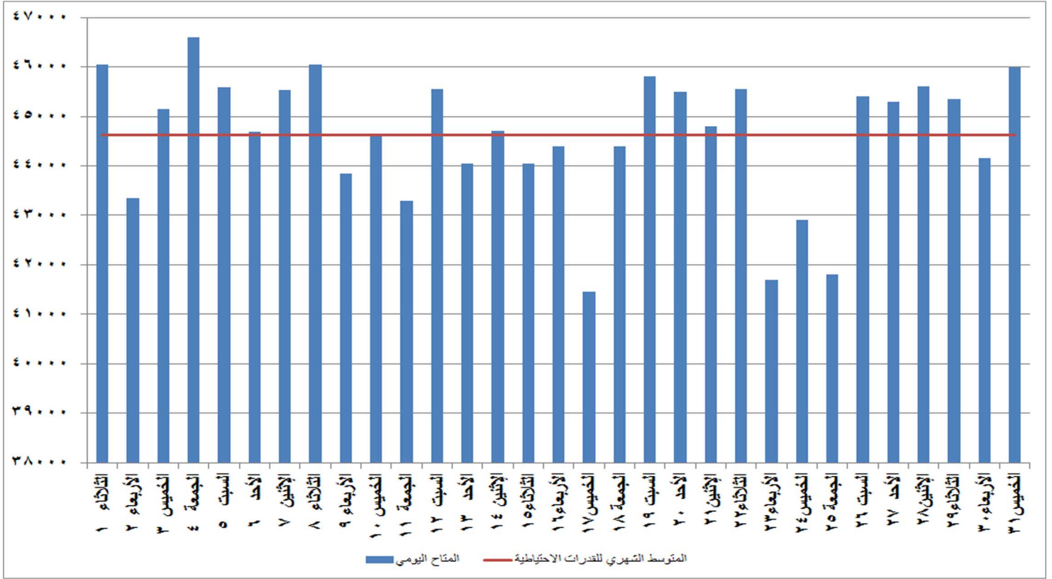
شكل (٢٧) القدرات المتاحة يوميا والمتوسط الشهري للقدرة الاحتياطية خلال شهر أكتوبر ٢٠١٩
