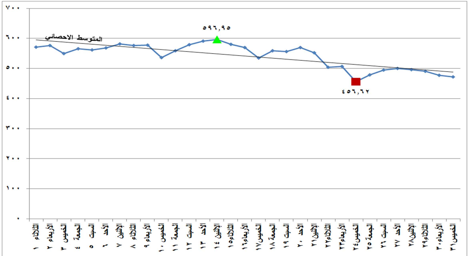
شكل (١٥) إجمالي الطاقة الكهربائية المنتجة من كل المصادر الأولية خلال شهر أكتوبر ٢٠١٩
