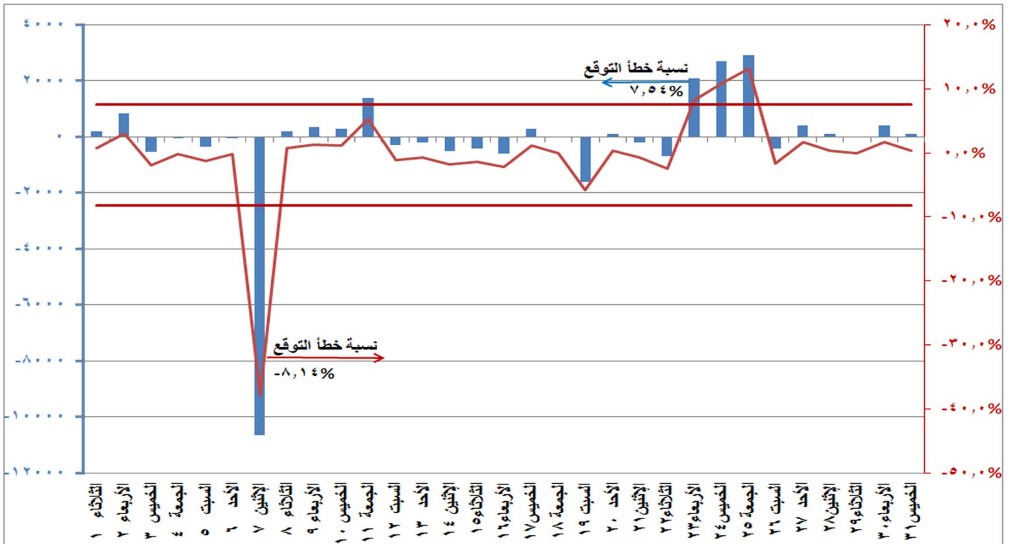
شكل (١٠) الفرق بين الحمل الأقصى المتوقع والمسجل فعليا ونسبة الفرق إلى الحمل المسجل فعليا خلال شهر أكتوبر ٢٠١٩
