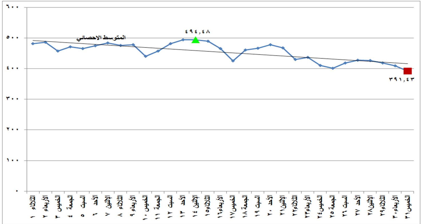
شكل (١٧) الطاقة الكهربائية المنتجة من الغاز الطبيعي خلال شهر أكتوبر ٢٠١٩
