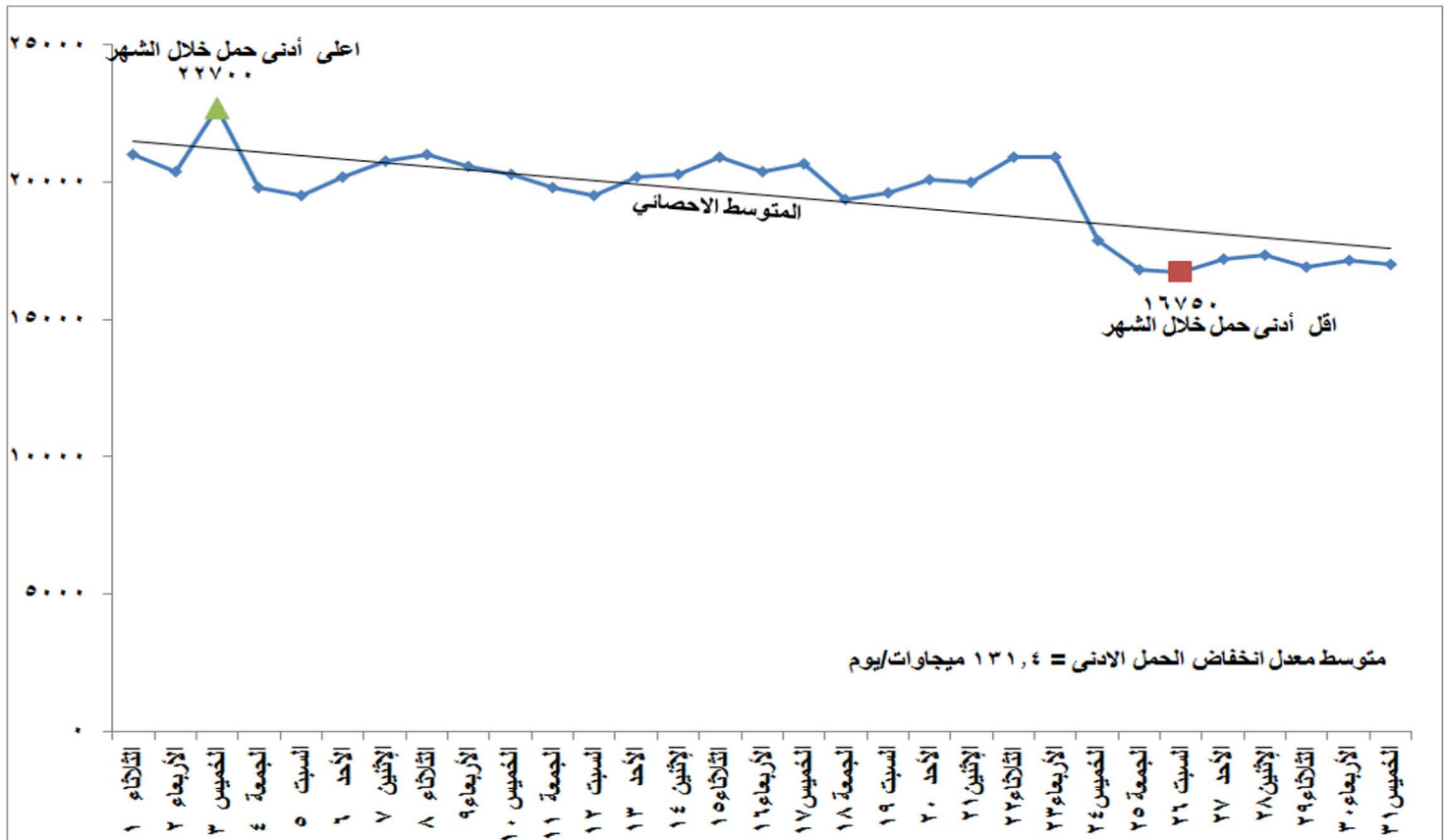
شكل (٢) تطور الحمل الادنى اليومي خلال شهر أكتوبر ٢٠١٩
