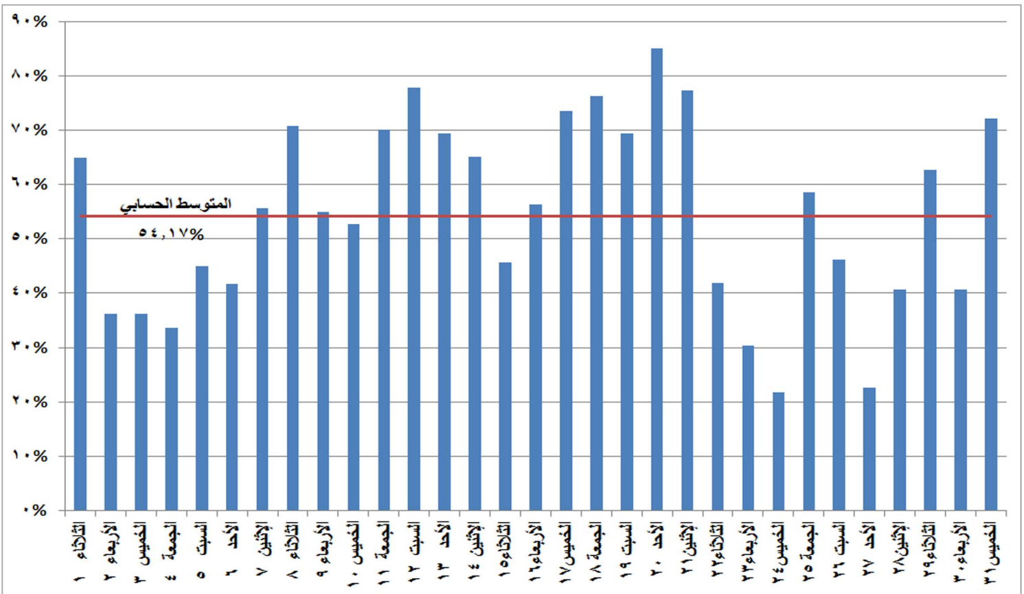
شكل (٢٢) نسب التغير في استخدام المصادر غير الحرارية في إنتاج الطاقة الكهربائية خلال شهر أكتوبر ٢٠١٩ مقارنة بالشهر المماثل من العام السابق
