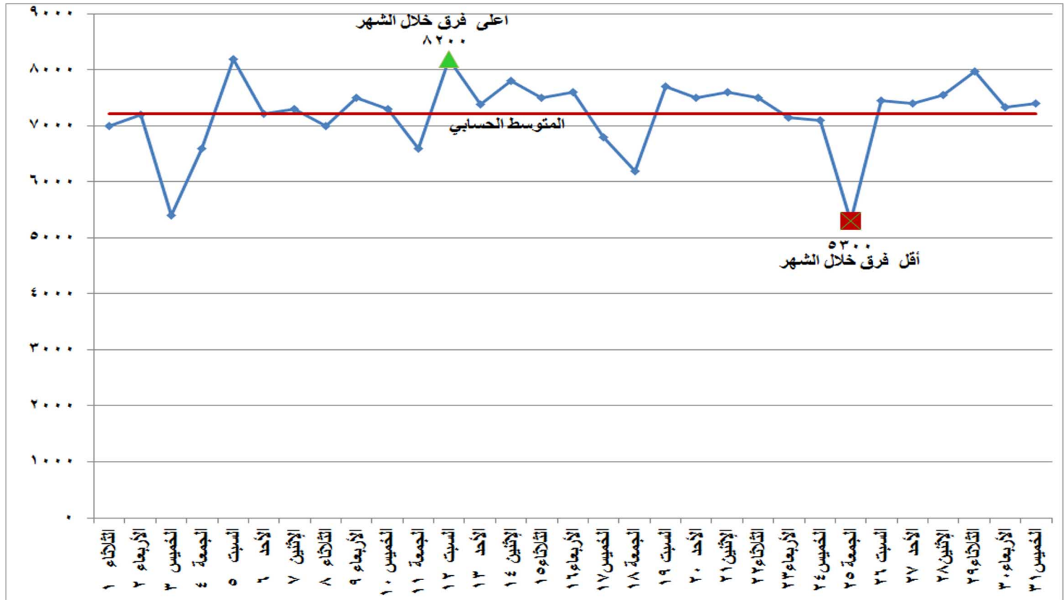
شكل (٣) الفرق بين أقصى وأدنى حمل خلال شهر أكتوبر ٢٠١٩
