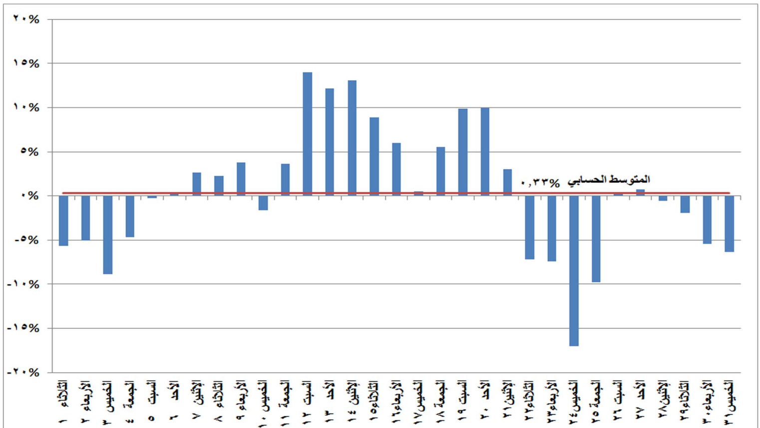
شكل (١٥) إجمالي الطاقة الكهربائية المنتجة من كل المصادر الأولية خلال شهر أكتوبر ٢٠١٩
