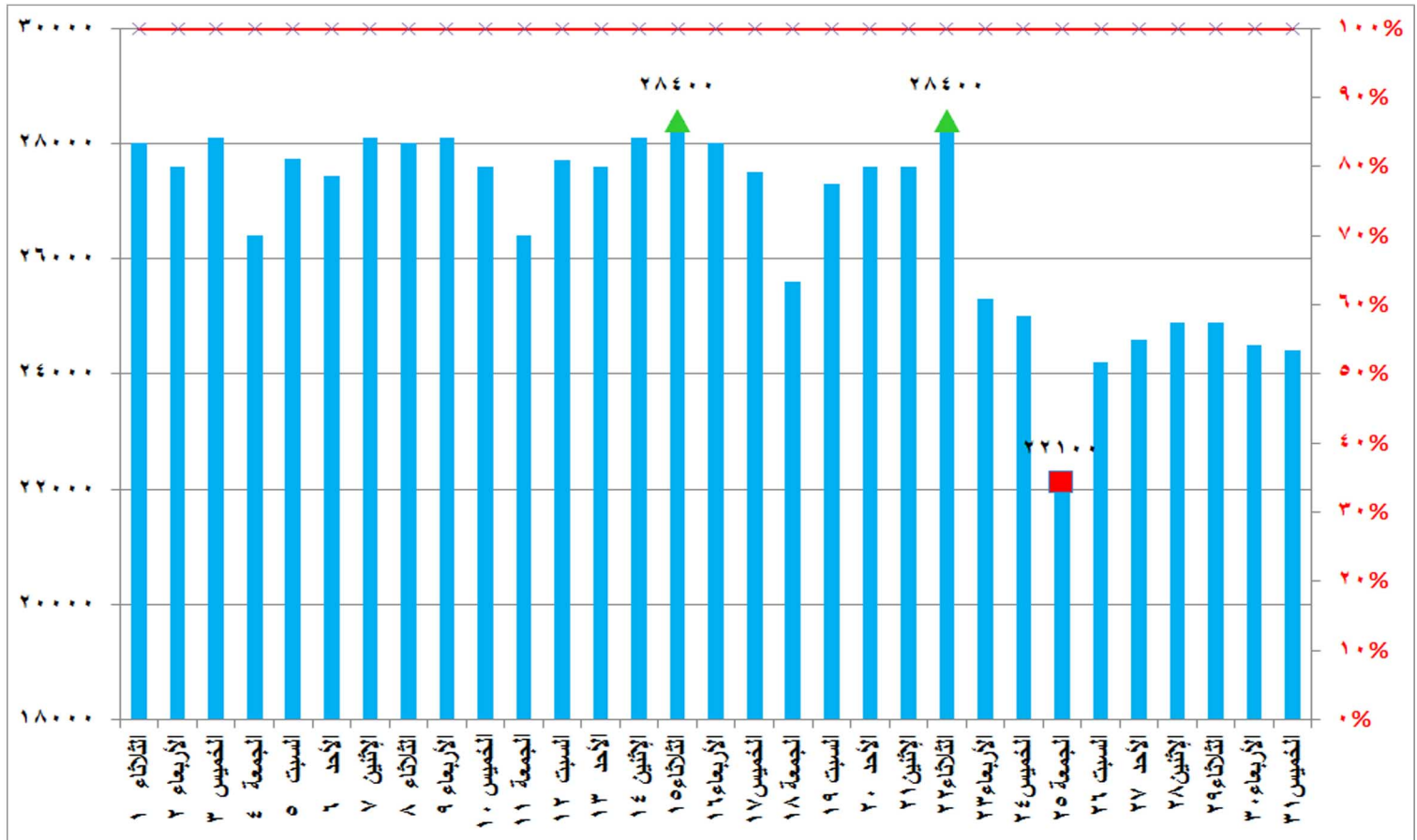
شكل (٥) قدرات الانتاج المتاحة ونسبتها للحمل الأقصى خلال شهر أكتوبر ٢٠١٩
