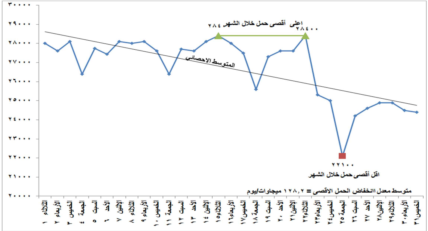
شكل (١) تطور الحمل الاقصى اليومي خلال شهر أكتوبر ٢٠١٩
