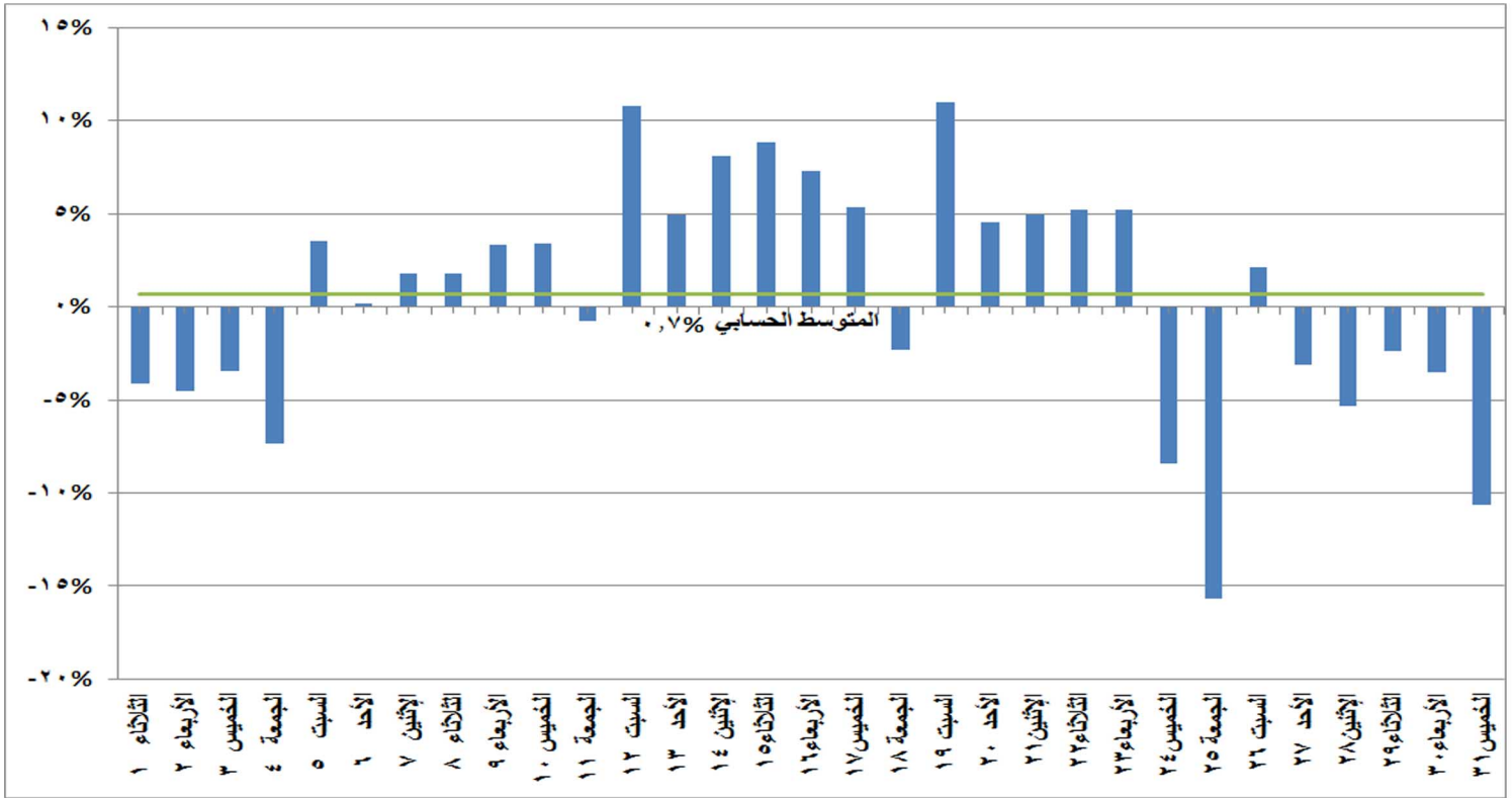
شكل (٩) النسب المئوية للتغير في الحمل الاقصى خلال شهر أكتوبر ٢٠١٩ مقارنة باليوم المماثل من العام الماضي
