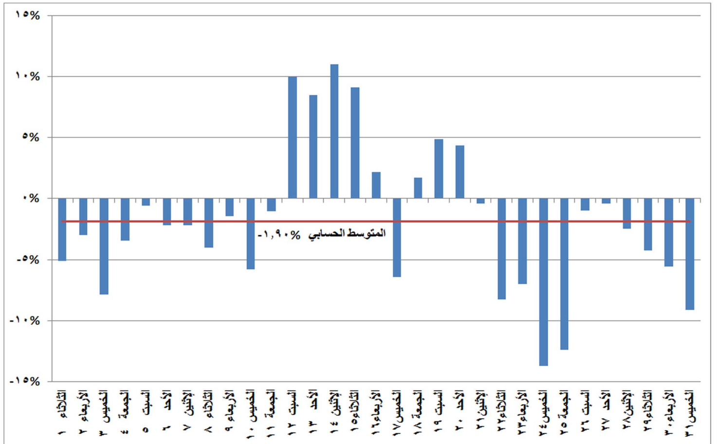
شكل (١٨) نسب التغير في استخدام الغاز الطبيعي في إنتاج الطاقة الكهربائية خلال شهر أكتوبر ٢٠١٩ مقارنة بالشهر المماثل من العام السابق
