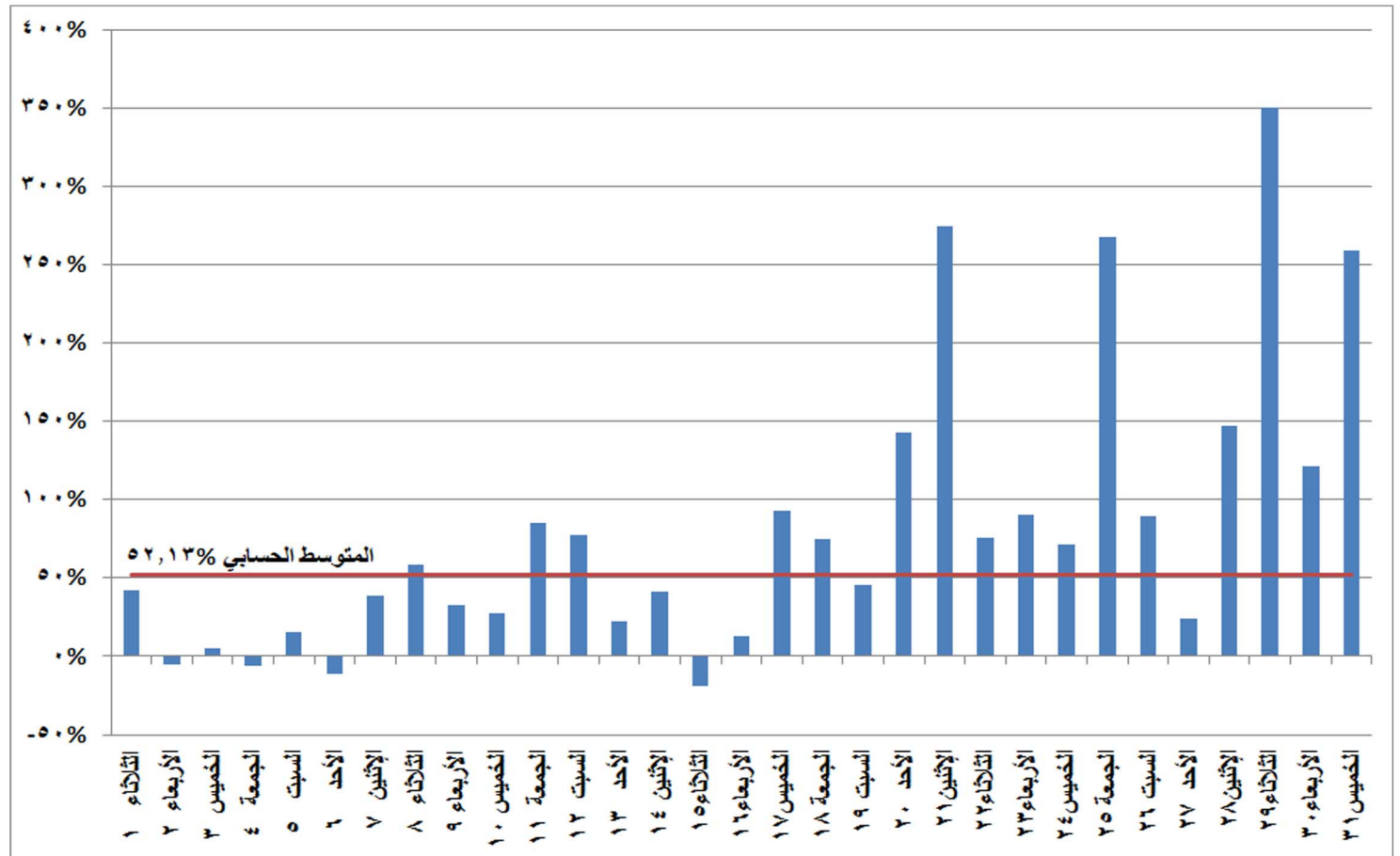
شكل (٢٦) نسب التغير في استخدام الرياح والشمس في إنتاج الطاقة الكهربائية خلال شهر أكتوبر ٢٠١٩ مقارنة بالشهر المماثل من العام السابق
