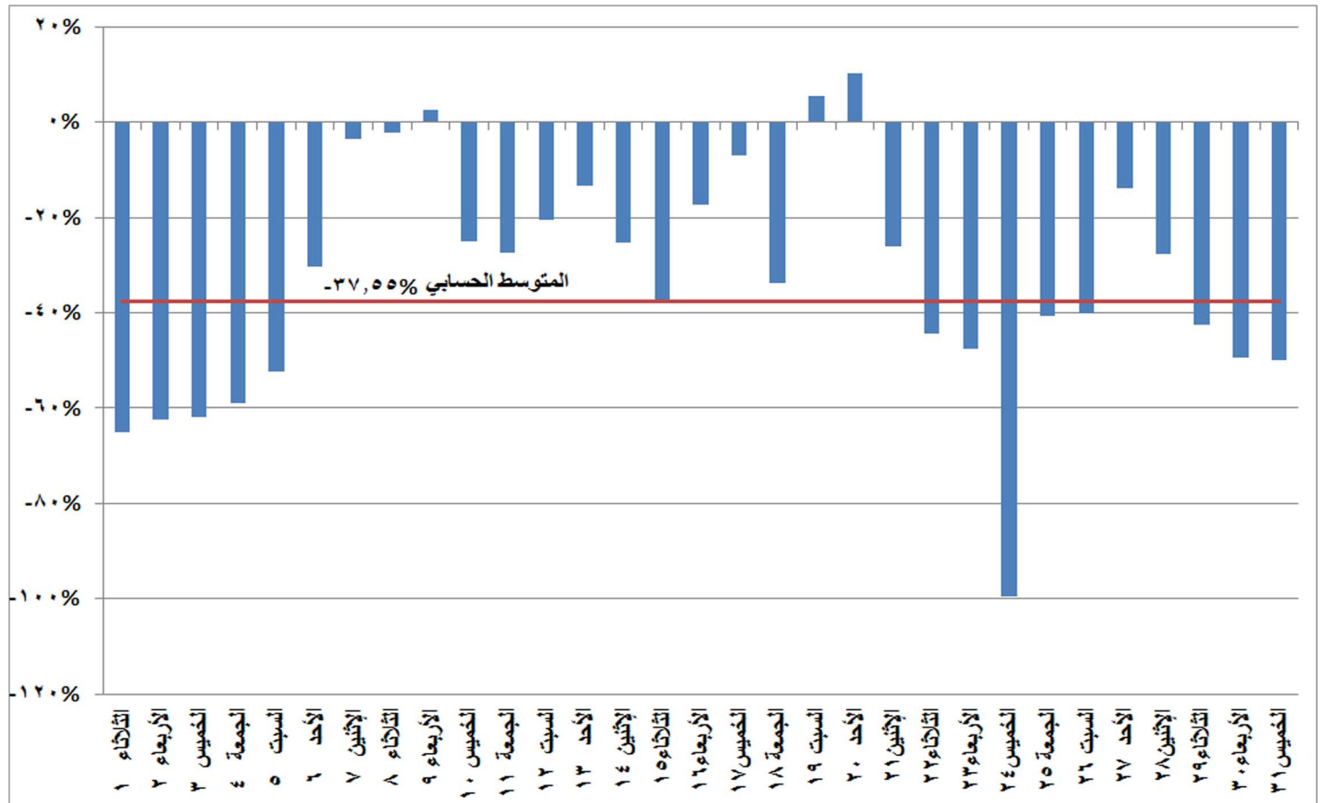
شكل (٢٠) نسب التغير في استخدام المازوت في إنتاج الطاقة الكهربائية خلال شهر أكتوبر ٢٠١٩ مقارنة بالشهر المماثل من العام السابق
