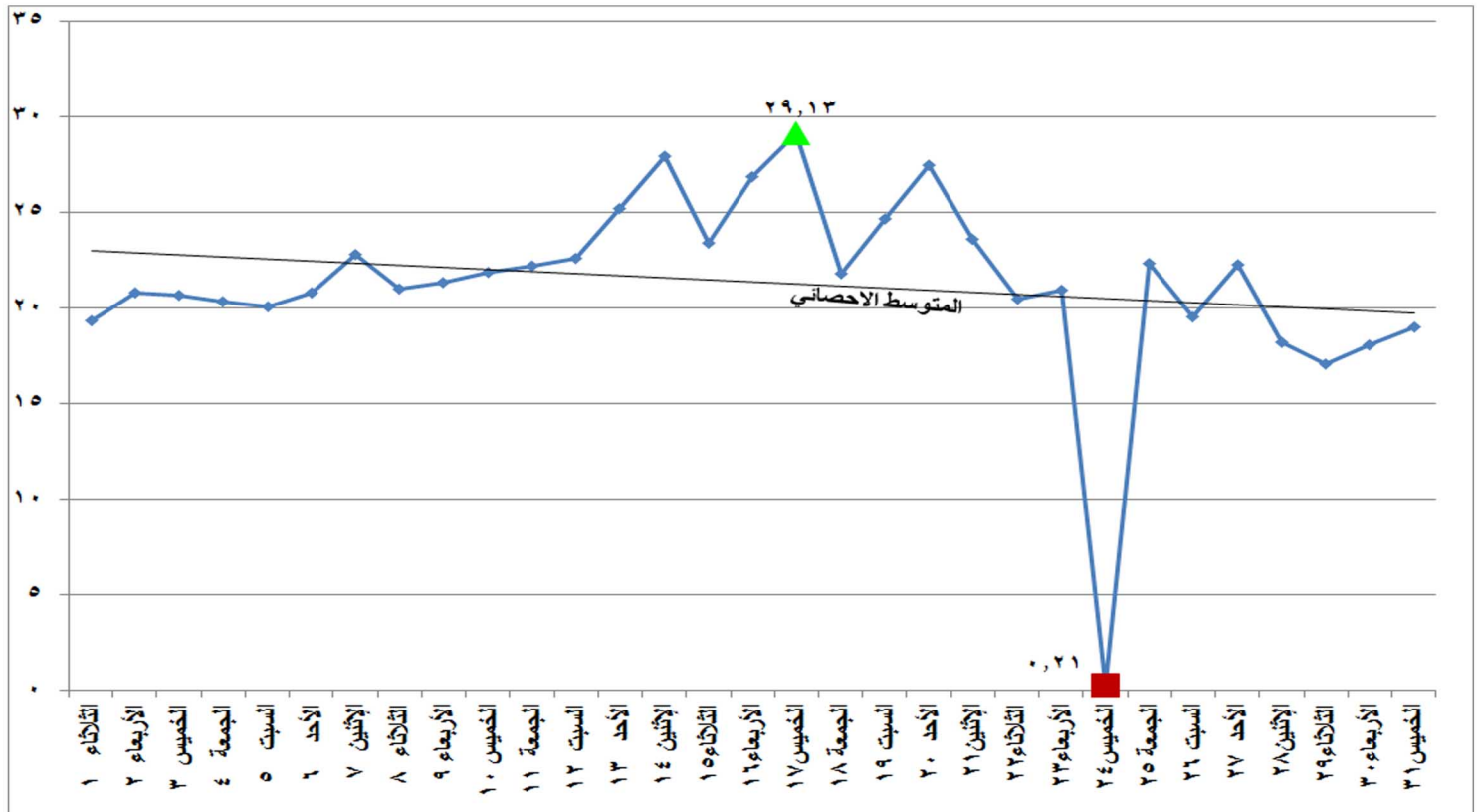
شكل (١٩) الطاقة الكهربائية المنتجة من المازوت خلال شهر أكتوبر ٢٠١٩
